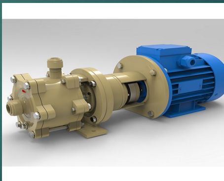
Электронасосные агрегаты типа ЭПНМ предназначены для питания автоматизированных котло-агрегатов, устанавливаемых на судах и плавсредствах с неограниченным районом плавания
